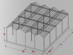
نقشه شماتیک نمای کلی از بخشی از سازه گلخانه و معیار های محاسباتی (بر عرض ۶ متر و ارتفاع ۲.۵ متر)
