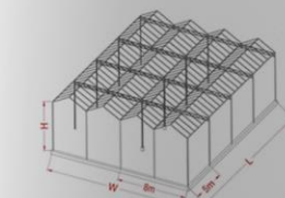
نقشه شماتیک نمای کلی از بخش از سازه گلخانه و دیوارهای طول (L)، عرض (W) و ارتفاع (H)
